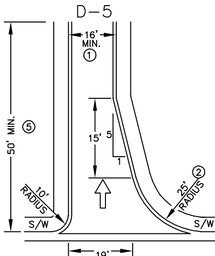
ONE WAY INGRESS (SEE MAG DTL 251)
